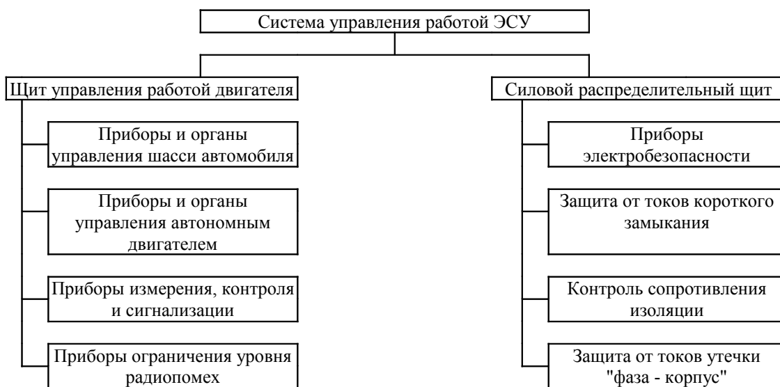
Структура системы управления работой ЭСУ АСА
